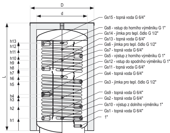
SCHÉMA AKUMULAČNÍHO ZÁSOBNÍKU O objemu 380-5000 lt
