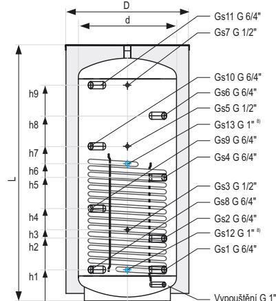
SCHÉMA AKUMULAČNÍHO ZÁSOBNÍKU o objemu 300-2000 lt
