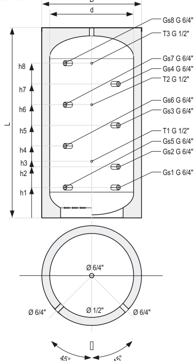
SCHÉMA AKUMULAČNÍHO ZÁSOBNÍKU o objemu 3000-5000 lt
