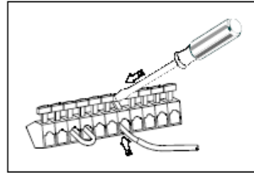
Obr. 3 – Upevnění kabelů do sverek
