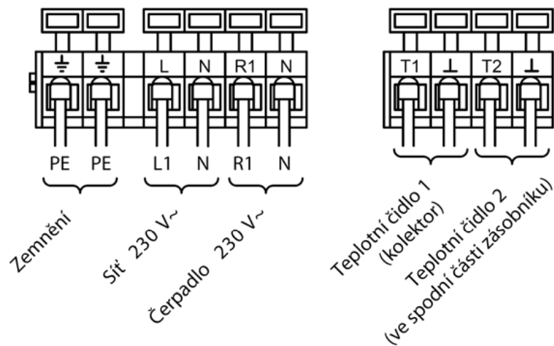
Obr. 4 – Schéma napojení na svorkovnici
