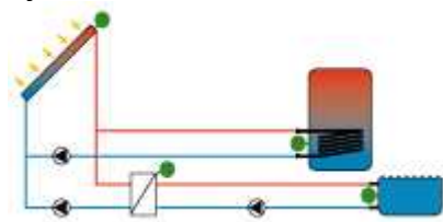
1x kolektorové pole, zásobník, bazén, externí výměník
