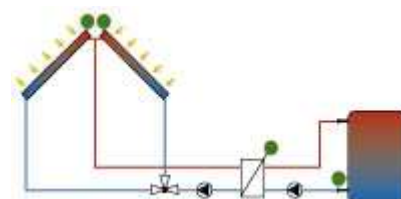
2x kolektorové pole, externí výměník
