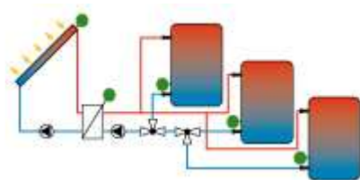
1x kolektorové pole, 3x zásobník, externí výměník
