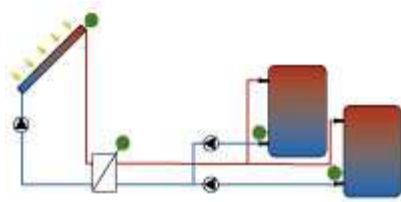
1x kolektorové pole, externí výměník, 2x zásobník
