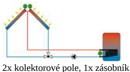
2x kolektorové pole, 1x zásobník
