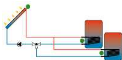
1x kolektorové pole, 2x zásobník
