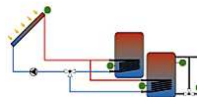
1x kolektorové pole, 2x zásobník, řízený obtok
