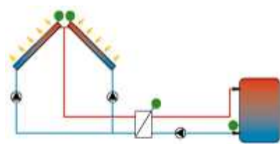
2x kolektorové pole, externí výměník
