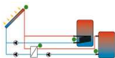
1x kolektorové pole, 2x zásobník, 1x externí výměník
