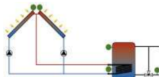
2x kolektorové pole, řízený obtok
