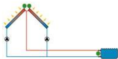
2x kolektorové pole, bazén
