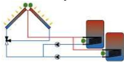
2x kolektorové pole, 2x zásobník
