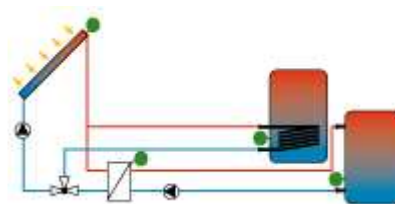
1x kolektorové pole, 2x zásobník, externí výměník
