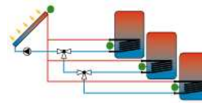
1x kolektorové pole, 3x zásobník
