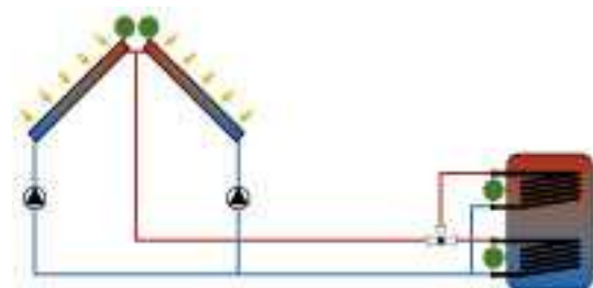
2x kolektorové pole, řízené nabíjení
