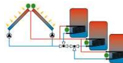
2x kolektorové pole, 3x zásobník
