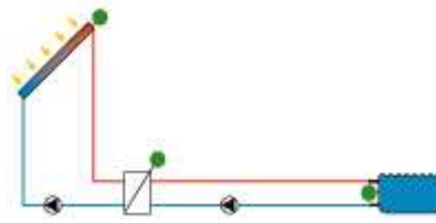
1x kolektorové pole, bazén, externí výměník
