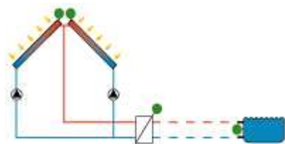
2x kolektorové pole, bazén, externí výměník
